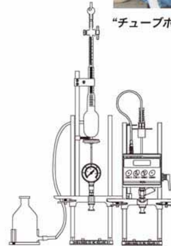
ガス飲料試作のための “パイロットプラント” (米 Zahm & Nagel 社)
